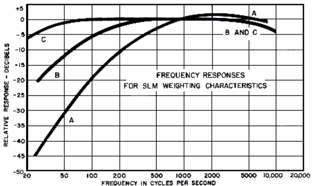
Figuur 2: verschillende wegingscurven voor dB(A) (dB(B)) en dB(C), met op de horizontale as de frequentie in Hz en op de verticale as de correctie in decibellen (zie ook noot 3, pg.5).
